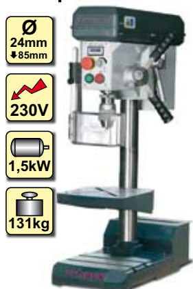
Opti B 24 H Vario
