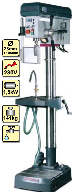
Opti B 28 H Vario
