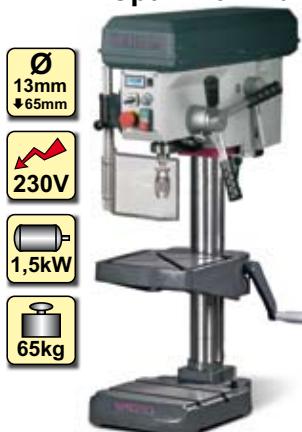
Opti B 16 H Vario
