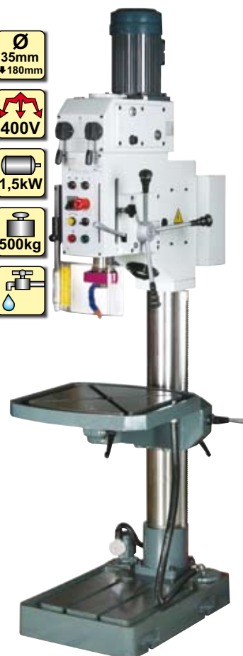
Opti B 40 GSP
