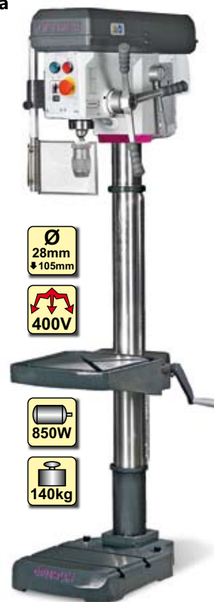
Opti B 28 H
