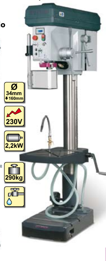
Opti B 34 H Vario
